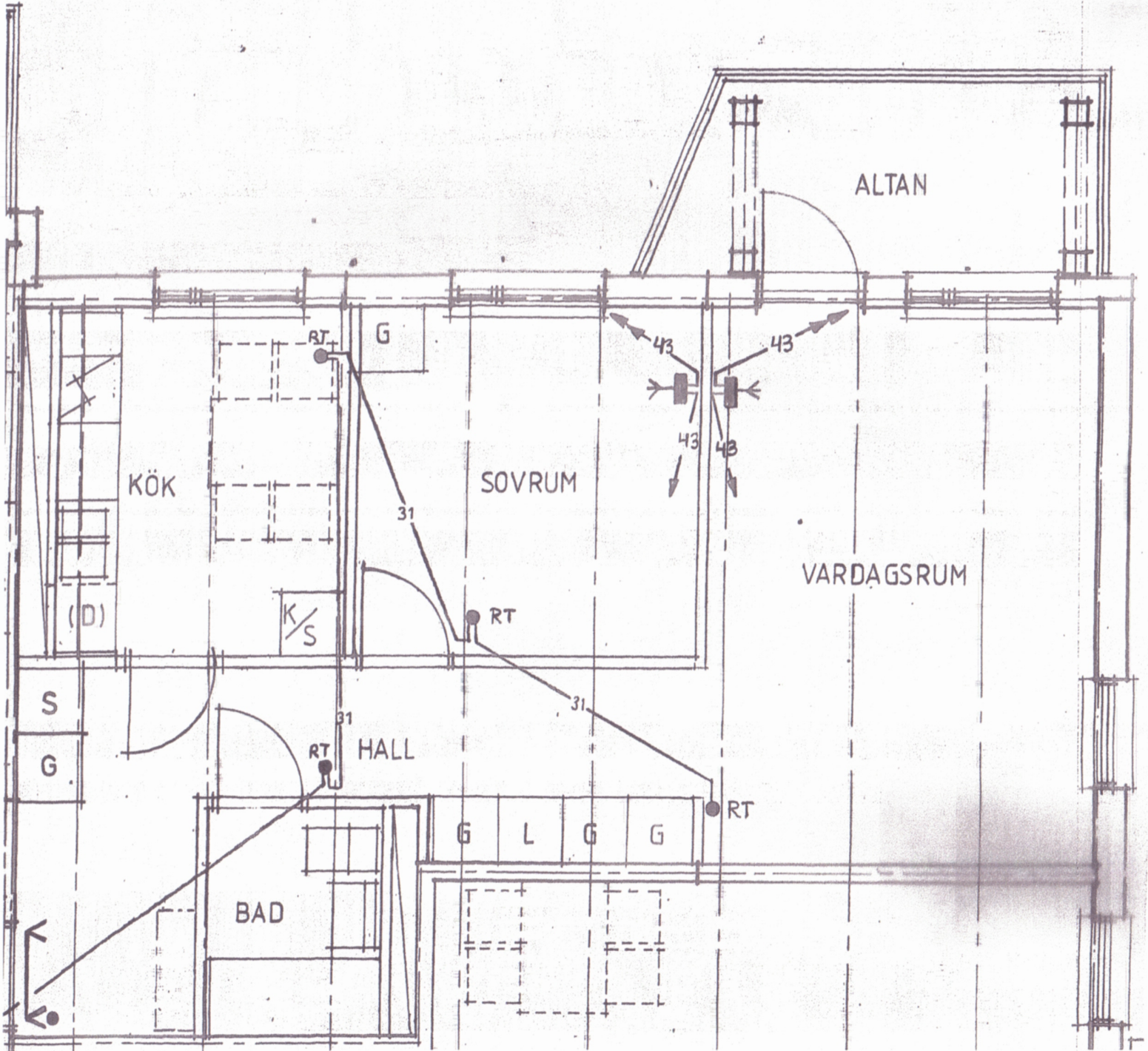
Tuvvägen 17 - 21 2 rum med kök Skala 1:50
